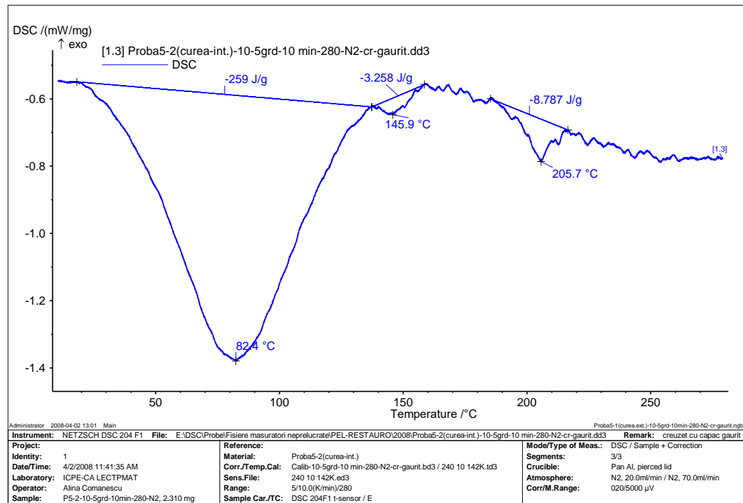
Fig. 1.13. Curba DSC pentru proba de piele P5-2
