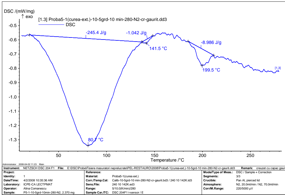
Fig. 1.12. Curba DSC pentru proba de piele P5-1
